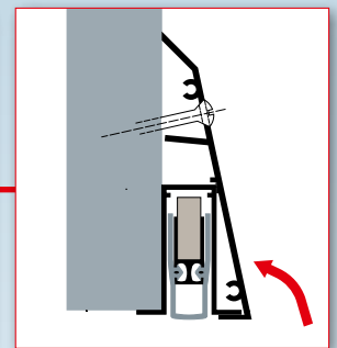
PLANET RF/FT MIT SOCKEL SEITLICH ZUR NACHRÜSTUNG
