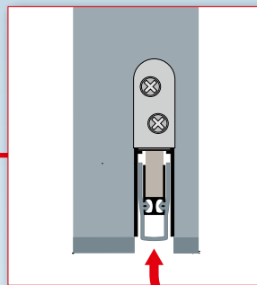
PLANET HS MIT RUNDLIPPE FÜR NORMALE BÖDEN
