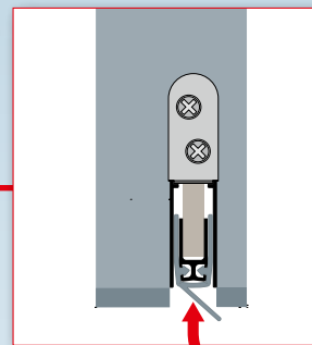
PLANET RH MIT SCHRÄGLIPPE FÜR WELLIGE BÖDEN
