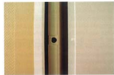
Nachrüst-Rauchschutzsystem „SRS-3“, „SD-1“ und „SRS-3-Clips“ an einer vorhandenen Stahl-Feuerschutztür
